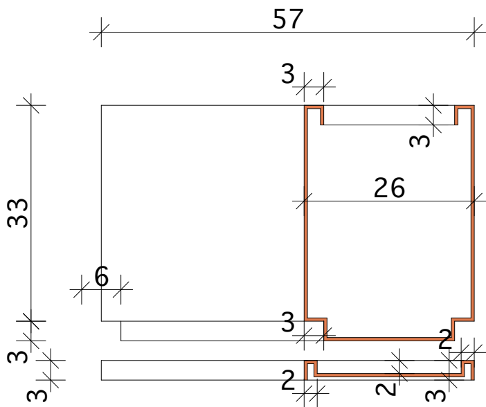
sez. A-A
